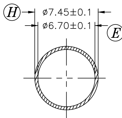
剖面A-A
