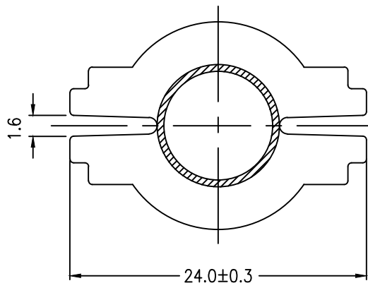
SEC. A-A
