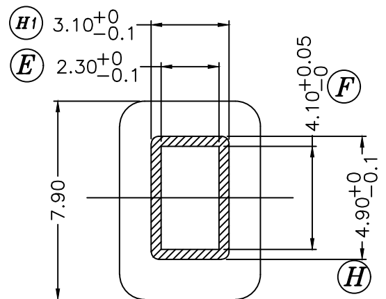
SEC A-A
