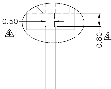
DETAIL A 2:1
