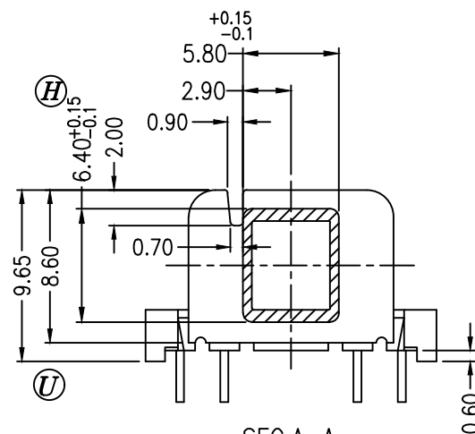
SEC.A-A
