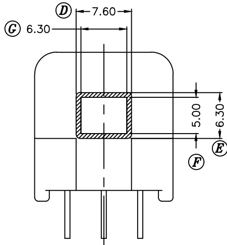
SEC A-A
