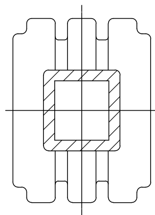
A-A SEC.
