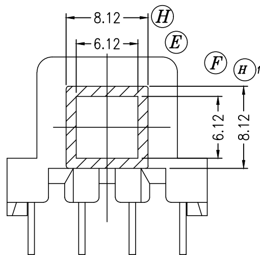
SEC.A-A
