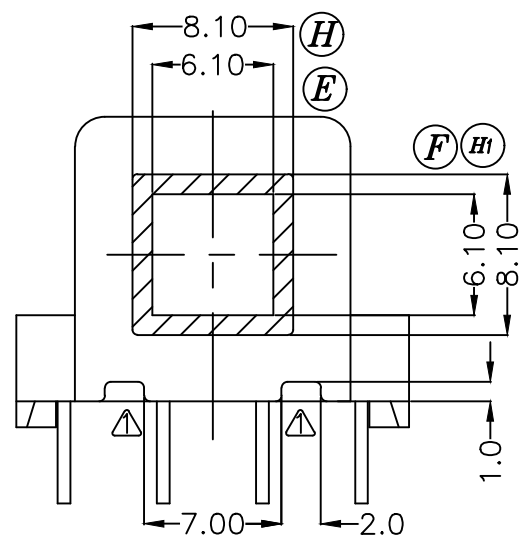
SEC.A-A
