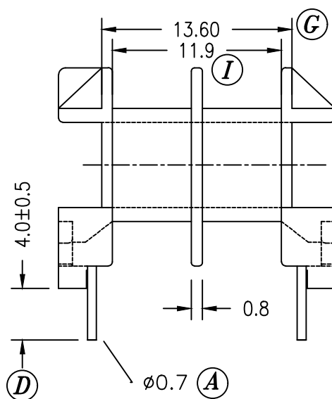
SEC.A-A
