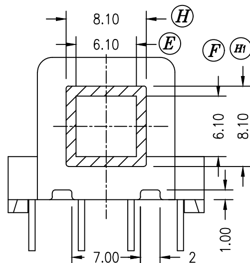
SEC.A-A
