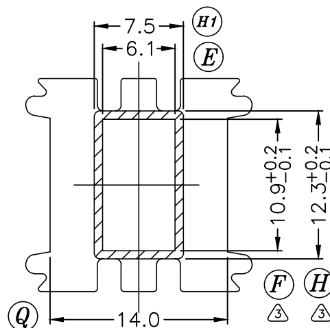
SEC.A-A
