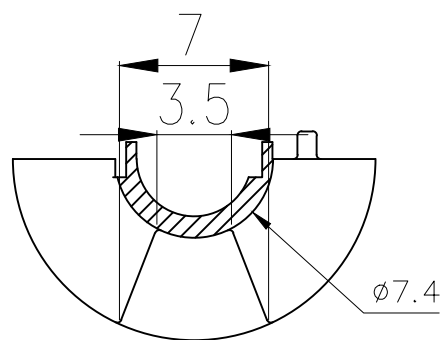
截面 A-A
