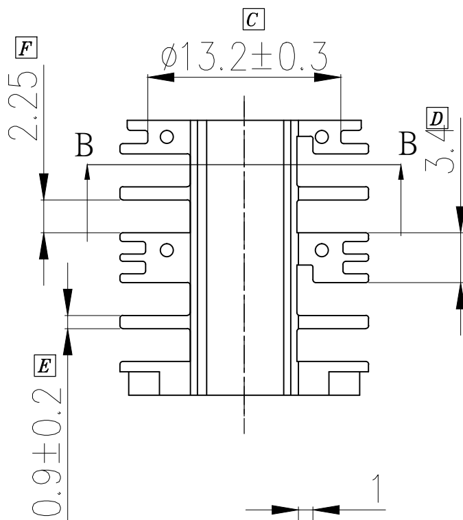
截面 A-A
