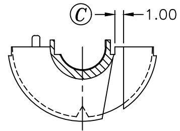
SEC.B-B
