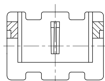
SEC. A-A
