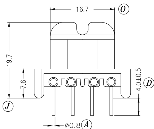
SEC.A-A
