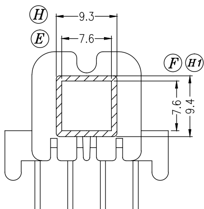
SEC.A-A
