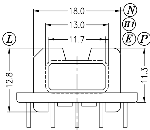
SEC. A-A
