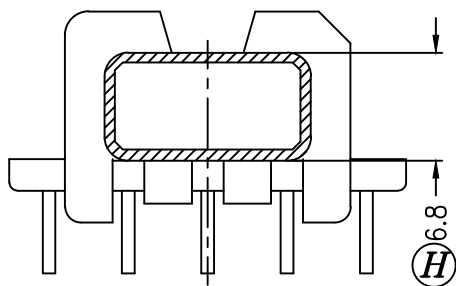
SEC. A-A
