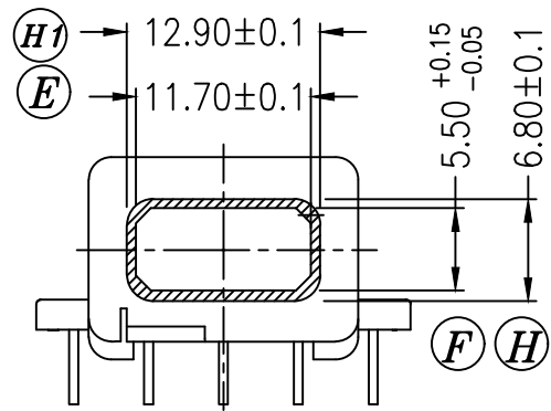
SEC. A-A
