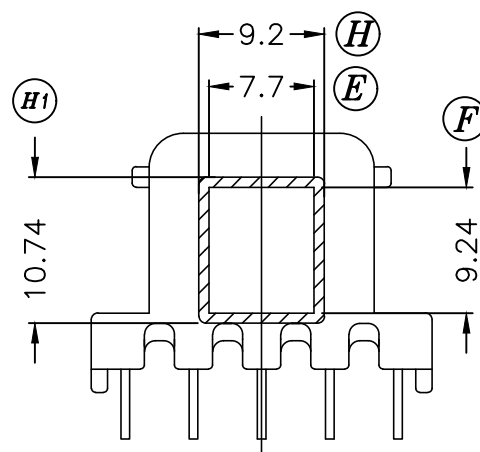
SEC.A-A
