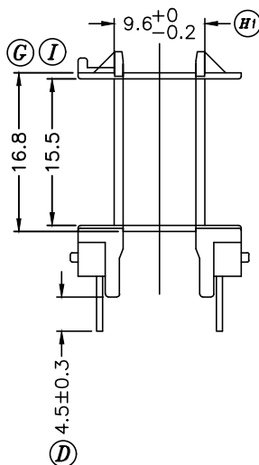
SEC.A-A
