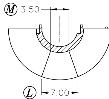
SEC.B-B
