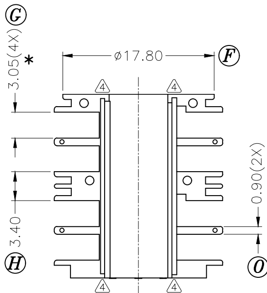
SEC.B-B
