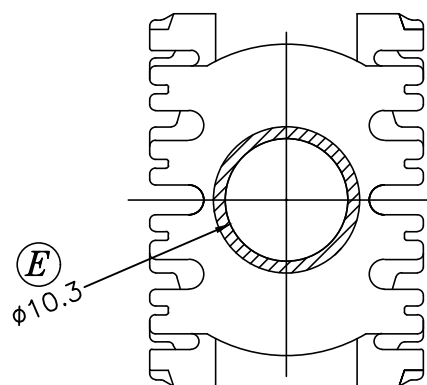
SEC. A--A
