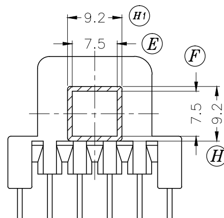
SEC.A-A
