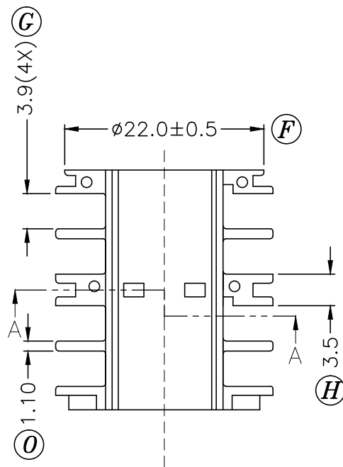
SEC.B-B
