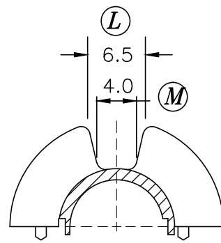
SEC.B-B
