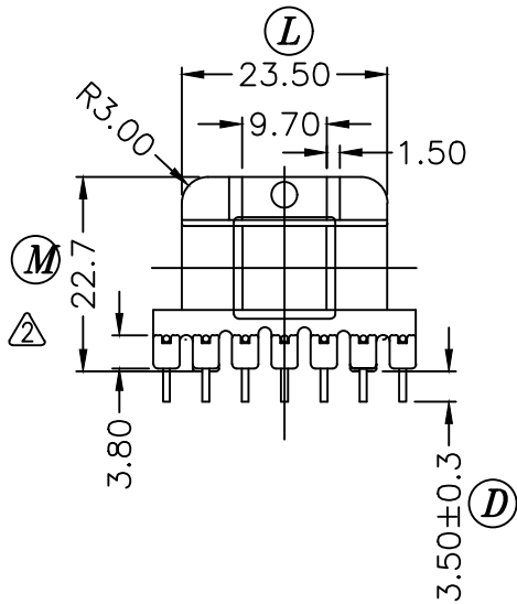
SEC. A-A
