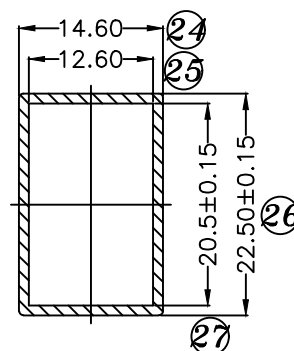
A-A SECTION
