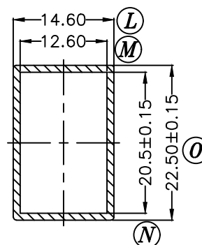
A-A SECTION
