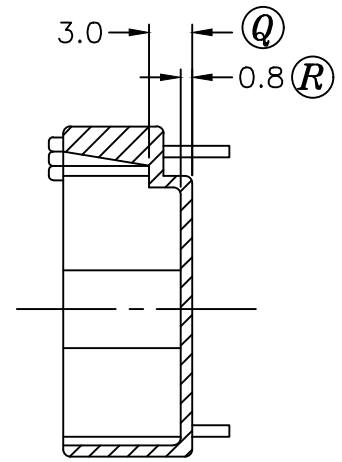
SEC.A-A
