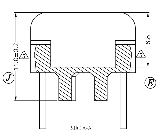
SEC A-A
