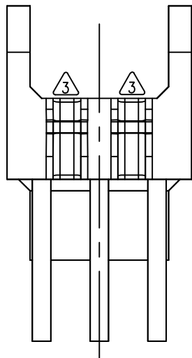
SEC A-A
