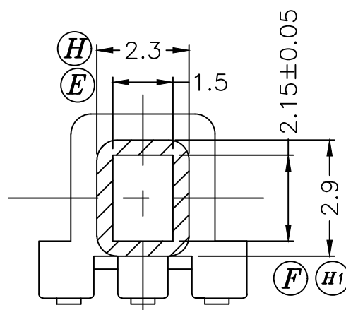
SEC. A-A
