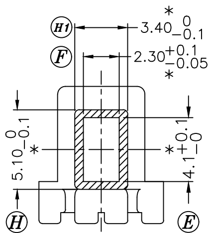
SEC A-A
