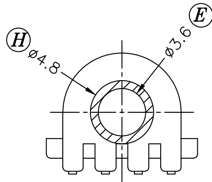
SEC. A-A
