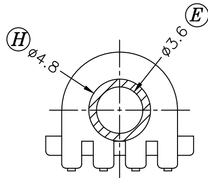
SEC. A-A
