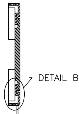
SEC.A-A
