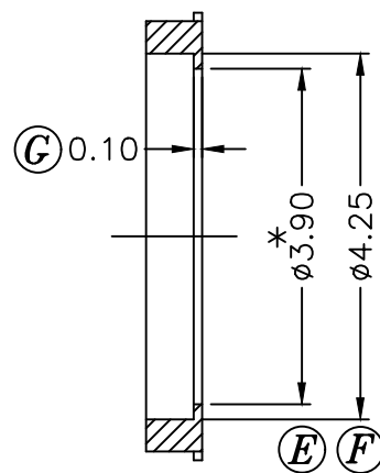
SEC.A-A
